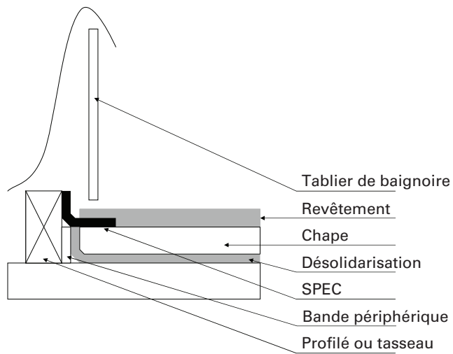
Figure 2 - Traitement de la réservation pour la pose d'une baignoire
